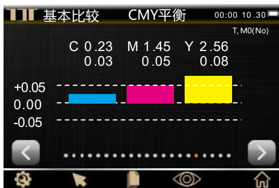
图50 基本比较的CMY平衡界面
